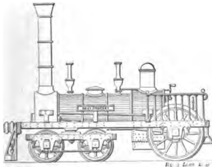
Fig. 80. Davy Crockett
