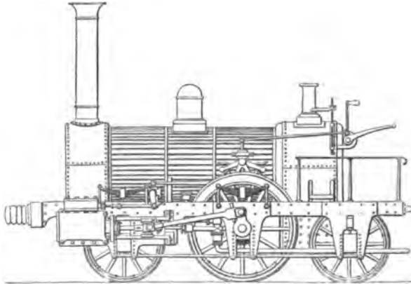
Fig. 17. Forrester, 1834
